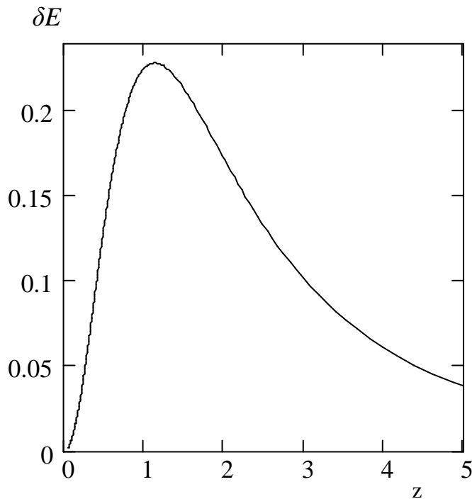
Fig. 11. \delta E = n \frac{dc_*^2 / dt_e}{H_0 c^2}
